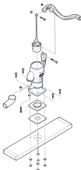
手押しポンプ部品図
