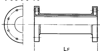
フランジタイプ
