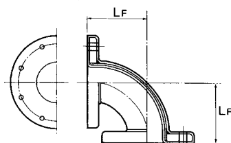
フランジタイプ
