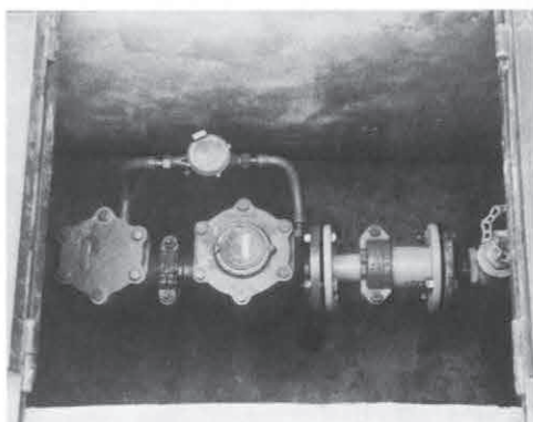
上水道メーター回り
