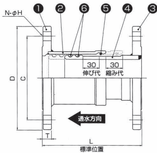
TST60/TST60-S 寸法
