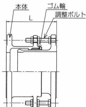
FF型寸法表
