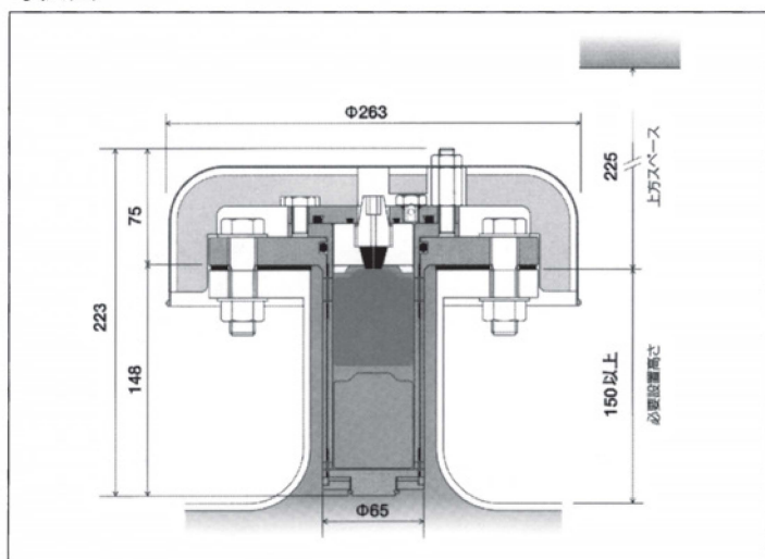
寸法図
