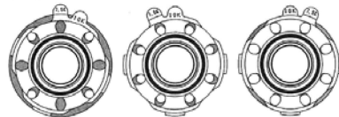
7.5Kフランジの場合 10Kフランジの場合 16Kフランジの場合
