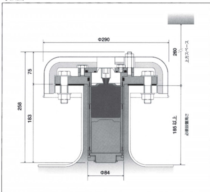
寸法図
