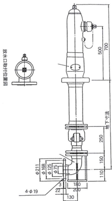
単 口（形式：CX1S-Z）
