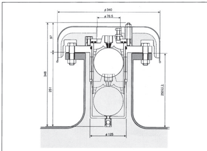
寸法図
