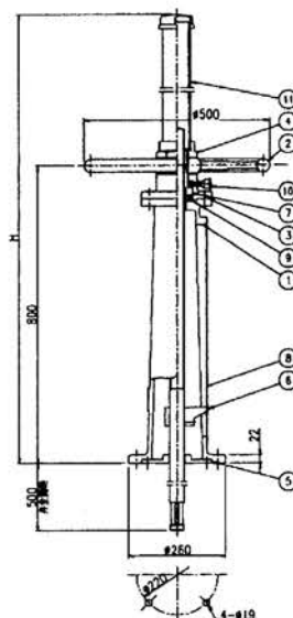
外ねじ開閉機 MFH-3
