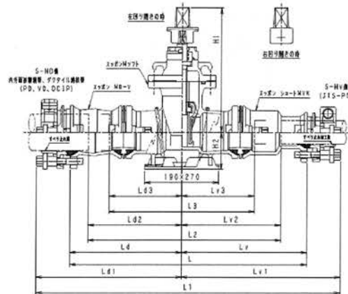
呼び径 定価 各部寸法 L L1 L2 L2' L2" L3 L3' L3" H1 H2 DCIP75 × JIS-P50 (弁体50) 148,370 397 550 279 51 228 253 38 215 300 85 呼び径 定価 各部寸法 L L1 L2 L3 Ld Ld1 Ld2 Ld3 Lv Lv1 Lv2 Lv3 H1 H2 DCIP75 × JIS-P50 (弁体75) 194,900 604 757 486 370 285 361 234 185 319 396 252 185 320 95
