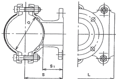
BV-P(硬質塩化ビニル管用) 寸法図 BS-P(鋼管用)
