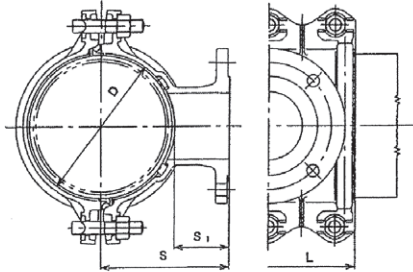
BCP-P(ダクタイル鋳鉄管・鋳鉄管) 寸法図
