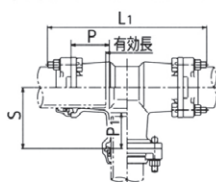
呼び径 40×40～200×200
