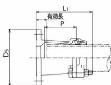
呼び径 50～200
