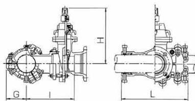
同口径ヤノT字管VK型
