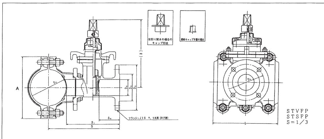
( 鋳鉄管用 \phi 75 \sim 200 \times \phi 75 \sim 200 ) ( STCPFP )
