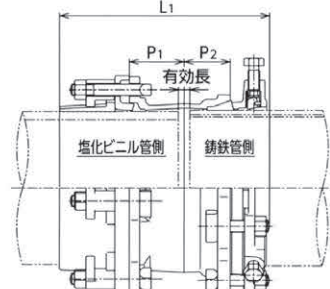
呼び径 250・300
