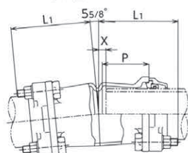
呼び径 50 ~ 200
