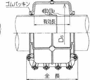
呼び径200～700
