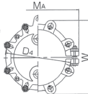
呼び径300~450
