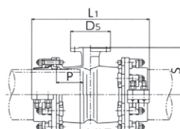
呼び径 250×75～300×200
