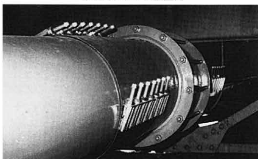
修理用クランプ設置例
