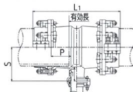
呼び径 250×75～300×300
