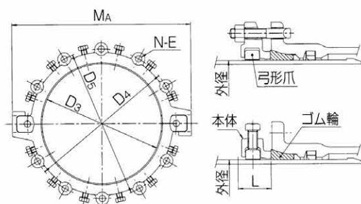
呼び径300~600
