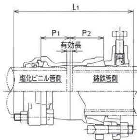
呼び径 75～200
