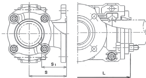
MP(配水用ポリエチレン管用) 寸法図
