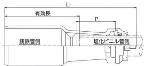
呼び径 75・100×50
