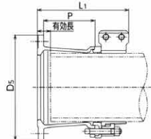
呼び径 250・300
