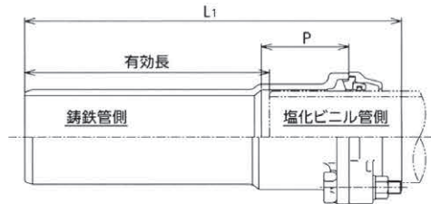
呼び径 75・100×50
