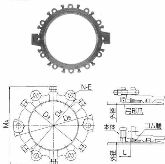
呼び径75~250
