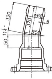
継ぎ輪
