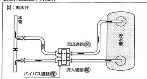
緊急弁作動説明図（平常時）
