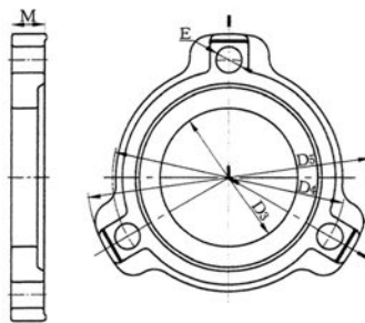
呼び径 350
