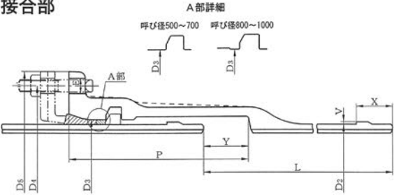
接合部
