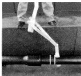
Step1 サイトコネクトを 挿し口部にセット
