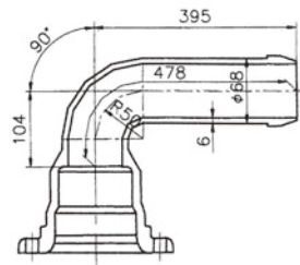
90° 曲管
