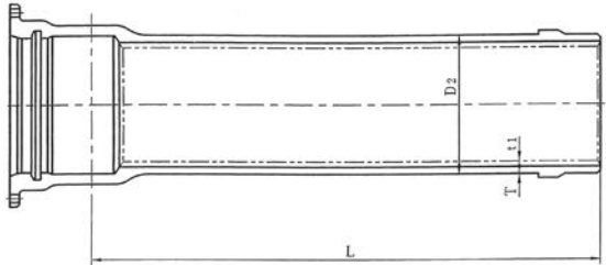
直部
