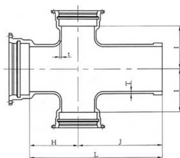
呼び径500～900
