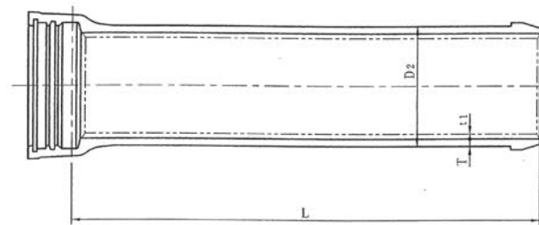
直部
