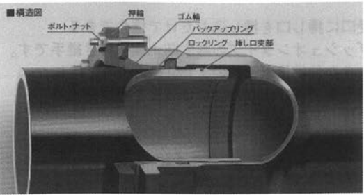
直部
