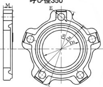
呼び径 350
