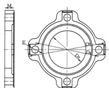
呼び径 400・450
