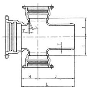
呼び径300～450
