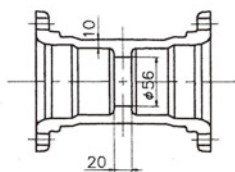
両受短管
