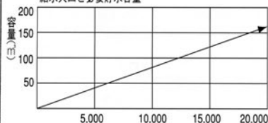
給水人口と必要貯水容量
