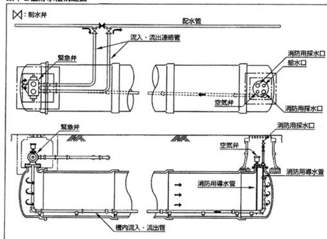
集中II型貯水槽構造図
