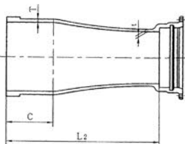
呼び径 500 ~ 1000
