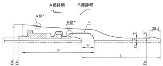
接合部
