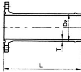
呼び径 75・100
