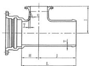
呼び径 300 ~ 450
