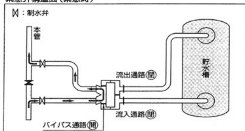
緊急弁作動説明図（緊急時）
