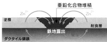
自己防食のメカニズム(イメージ)
