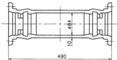
継ぎ輪
