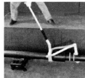
Step3 ハンドルを引いて管を 引き込み接合完了
