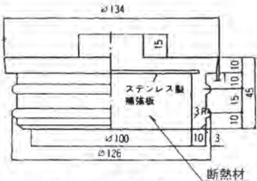
防水キャップ詳細図
