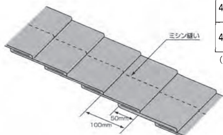
敷設例
